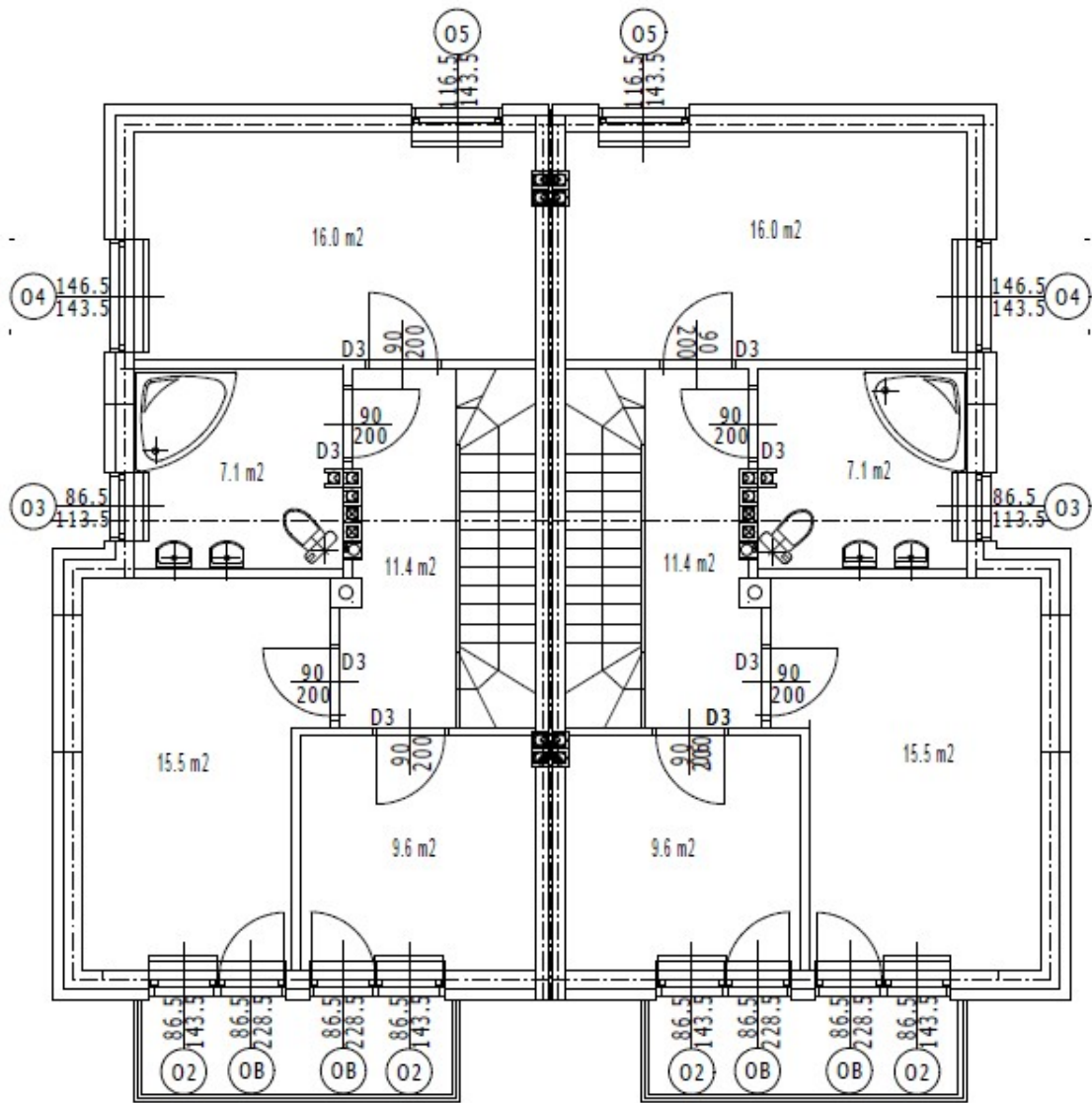
rzut poddasza
