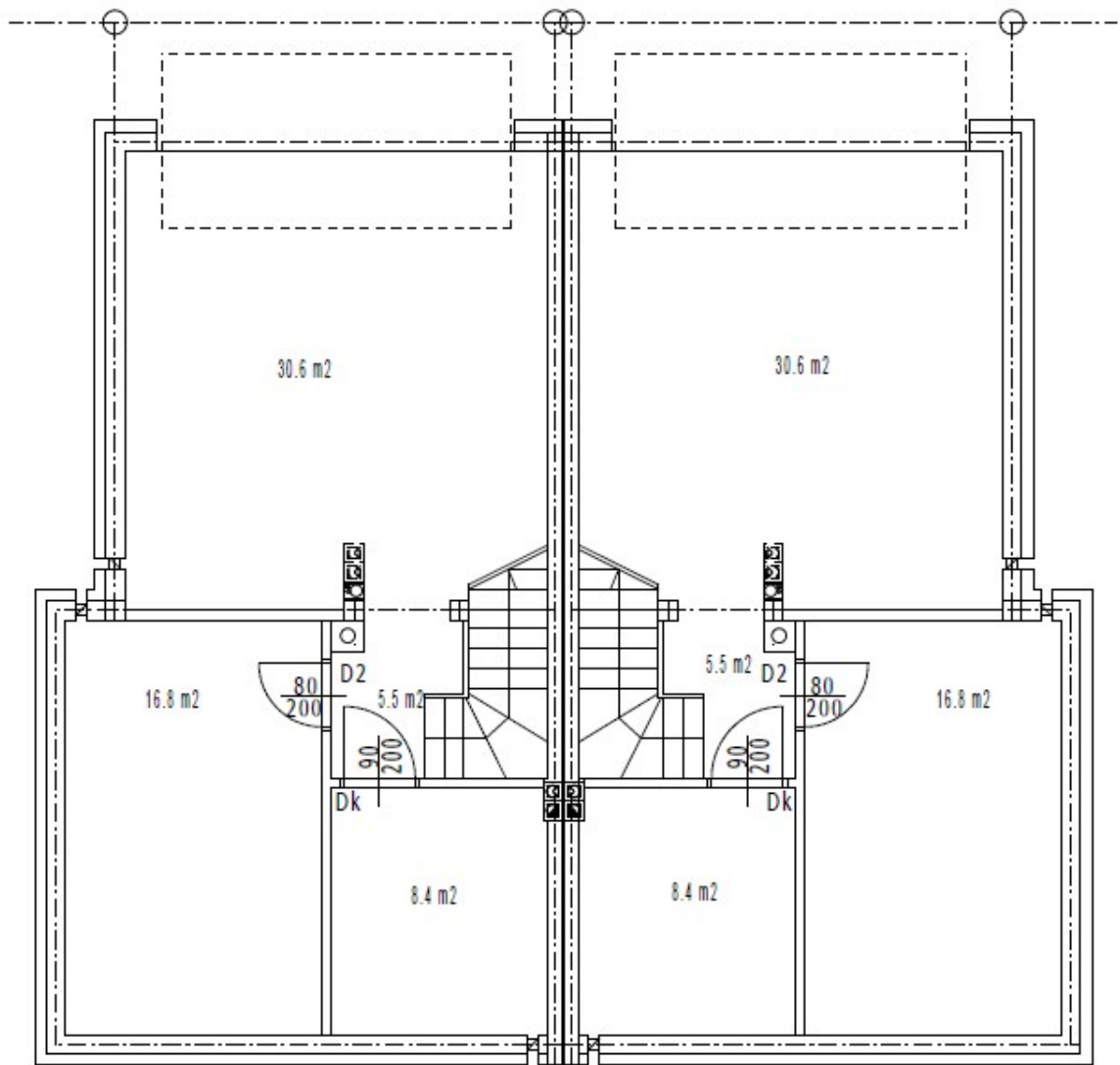
rzut piwnic
